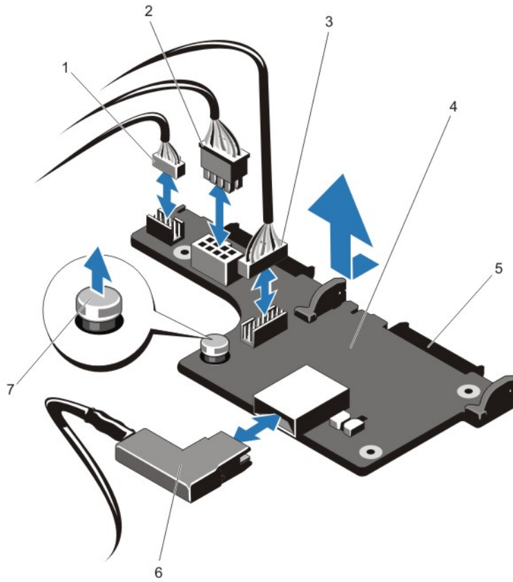
図 46. オプションの 2.5 インチ (x2) ハードディスクドライブバックプレーン (背面) の取り外しと取り付け
