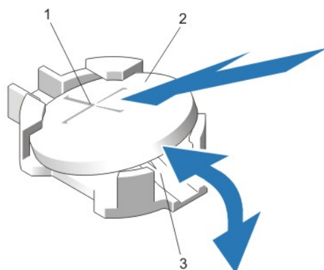
図 43. システムバッテリーの交換
