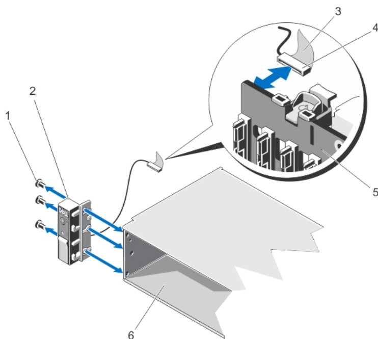
図 48. コントロールパネルの取り外しと取り付け
