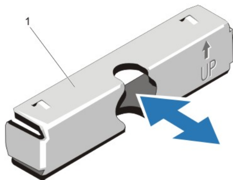
図 13. 2.5 インチハードドライブダミーの取り外しと取り付け（背面）
