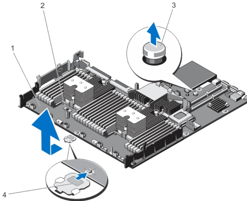
図 50. システム基板の取り外しと取り付け
