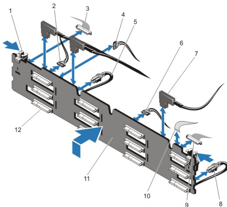
図 44.3.5 インチ (x12) SAS/SATA バックプレーンの取り外しと取り付け
