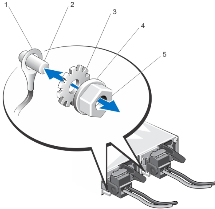
図 39. 保安接地線の編成と接続
