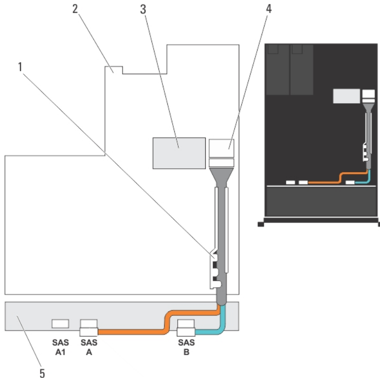
図 45. ケーブル接続図 — 3.5 インチ (x12) SAS/SATA バックプレーン
